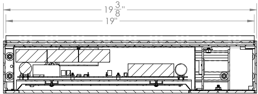
LONGITUDINAL VIEW
